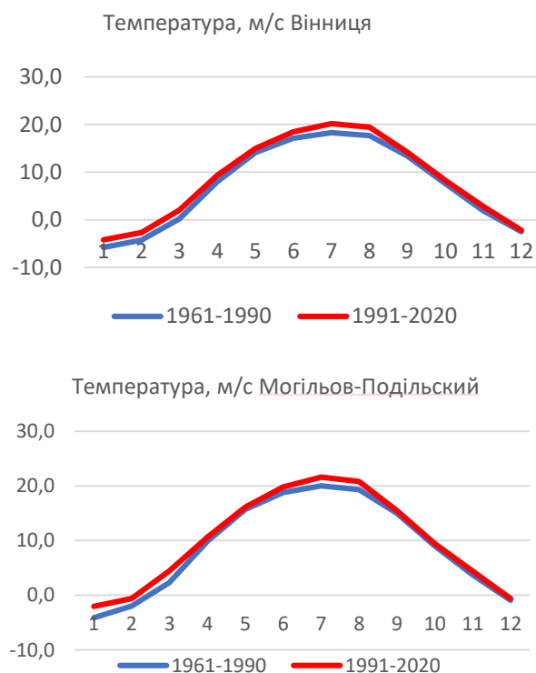
Рис. 3 – Порівняння річного ходу температури повітря за різні кліматичні періоди для метеостанцій Вінницької області
